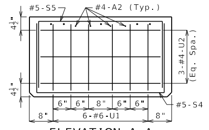
ELEVATION A-A
